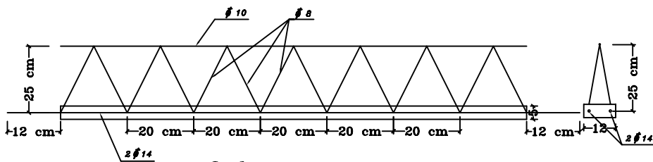
J-2 نمای تیرچه تیب
