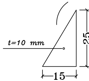
PL. (2) SC 1:10
