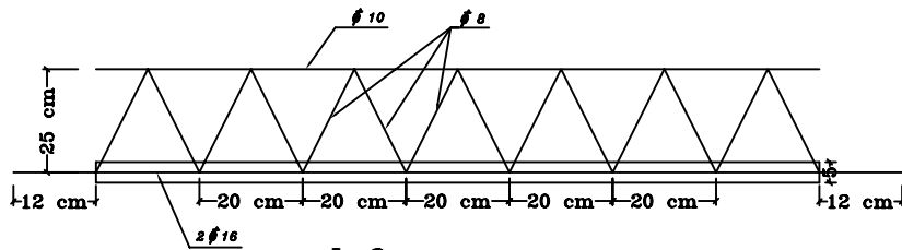
J-3 نمای تیرچه تیب
