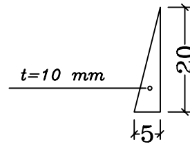
PL. (3) SC 1:10
