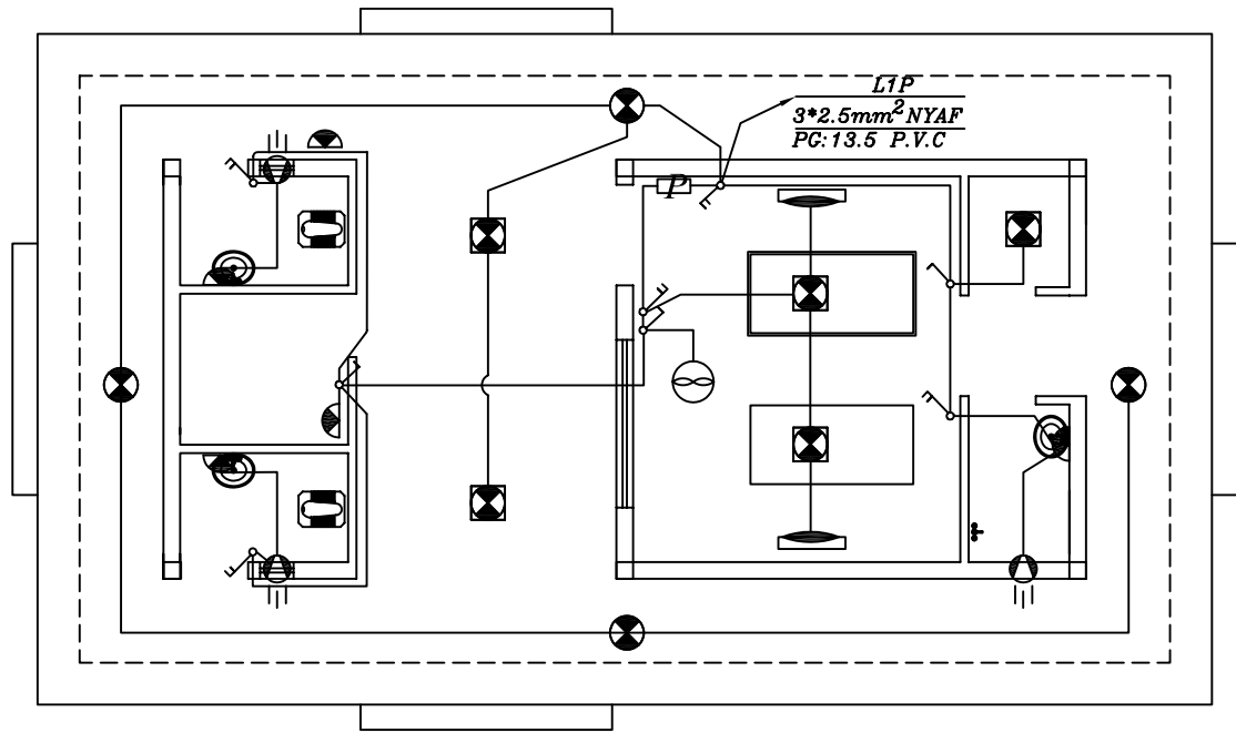
پلان روشنایی
