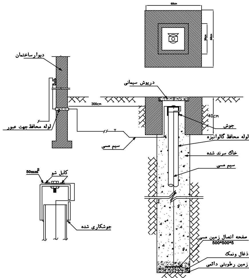
جزئیات چاه ارت
