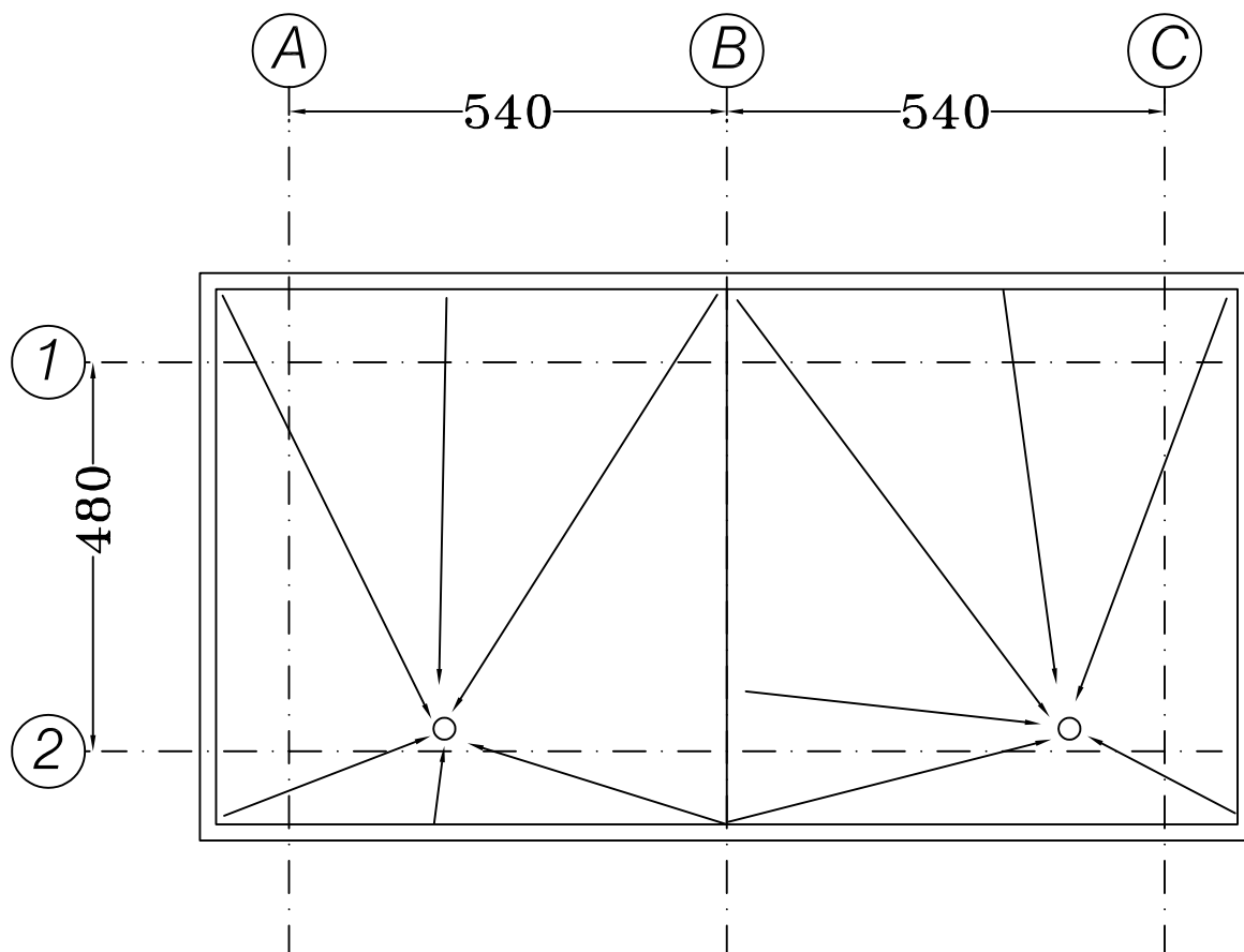
پلان شیب بندی
