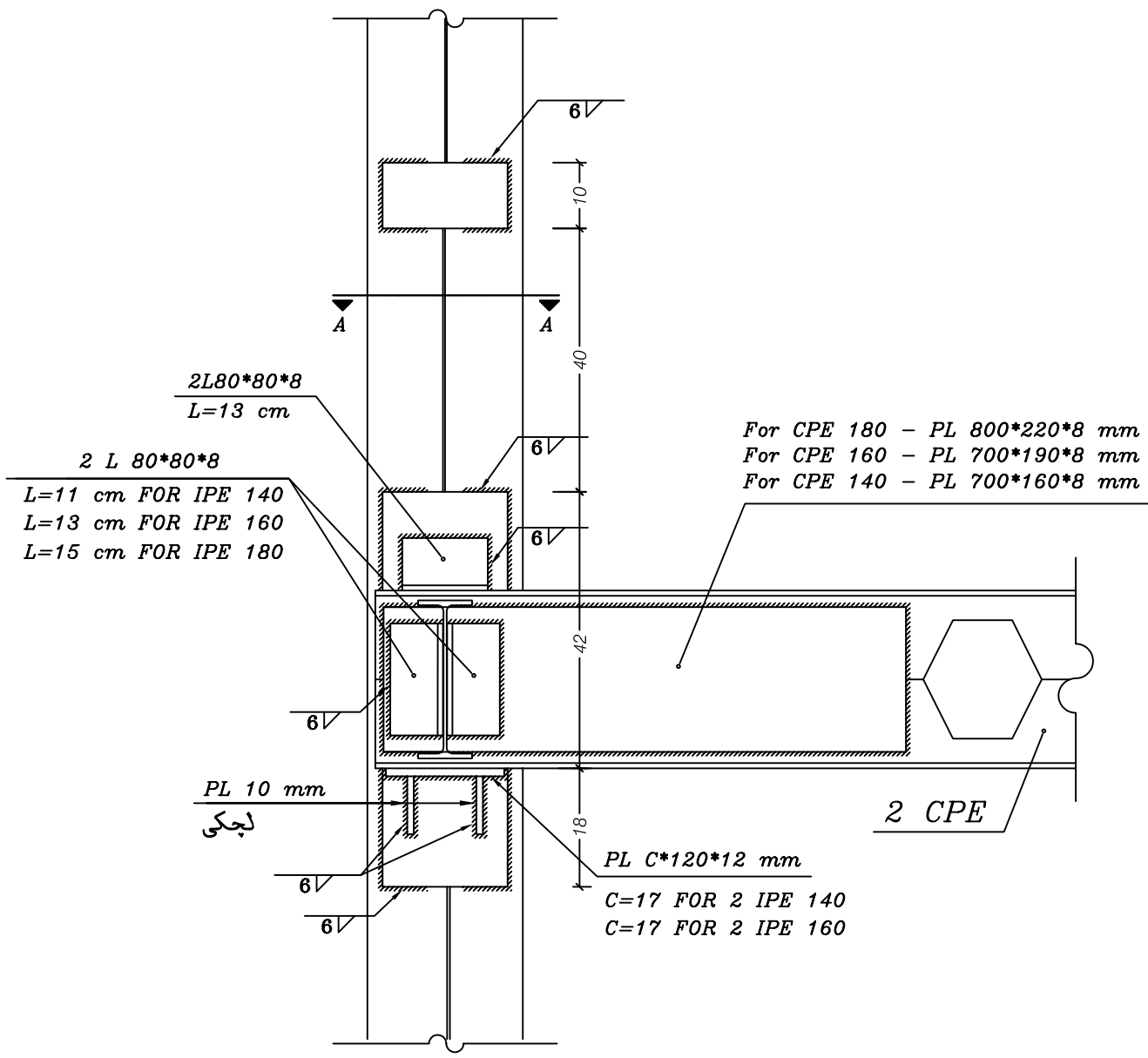
جزئیات محل عبور پلهای خورجینی از بر ستونهای کناری
